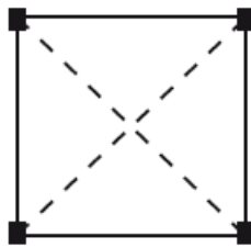
Схема "танца" с обменом местами
