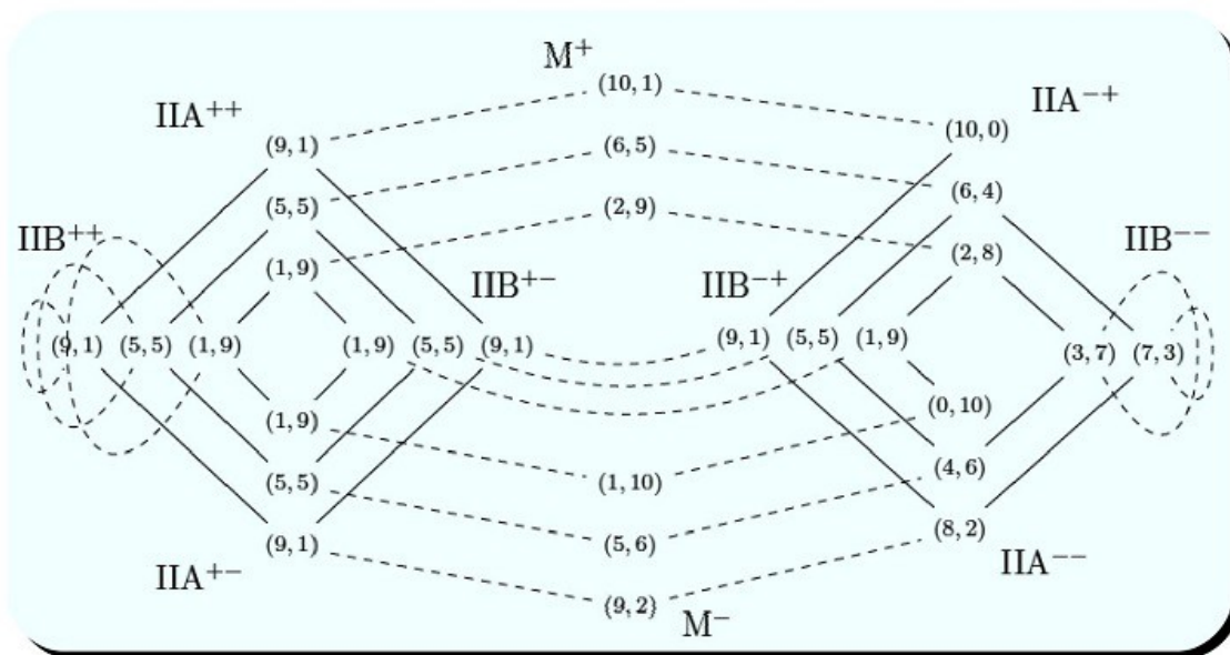
Сеть возможных сигнатур пространства-времени в M-теории и струнных теориях типа II
