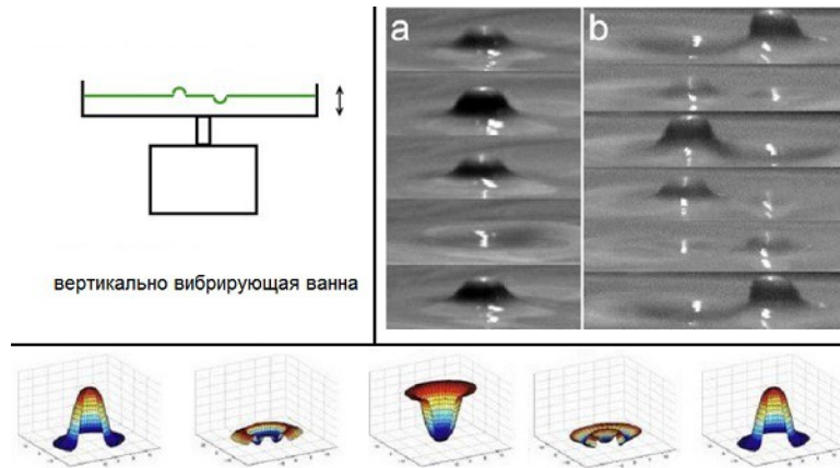
Классическая аналогия скалярных встряхиваний системы
